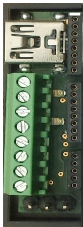
Aansluiting voor CV programmer
